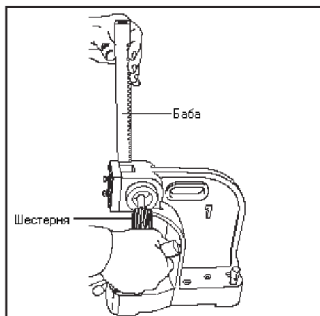
Рисунок 3. Позиционирование бабы
